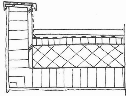
DETAIL DACHRANDABSCHLUSS MST 1:20
