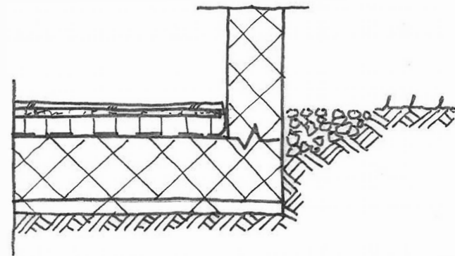
DETAIL BPL-WAND AUSSEN MST 1:20
